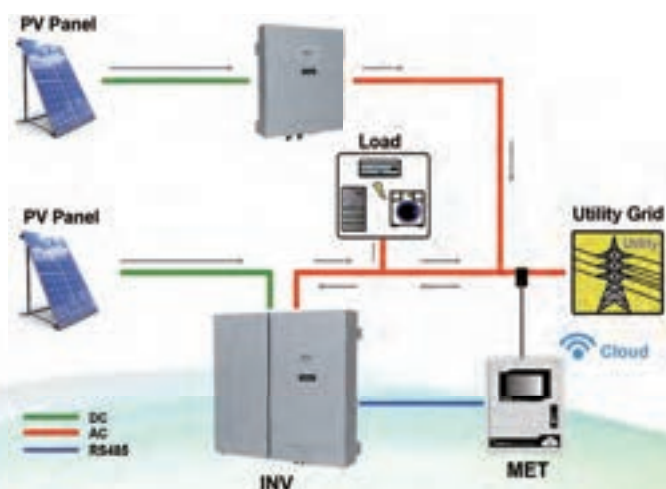
智慧型電網儲能系統 ESS (3~5kW) 電池 (2~12kWh)
